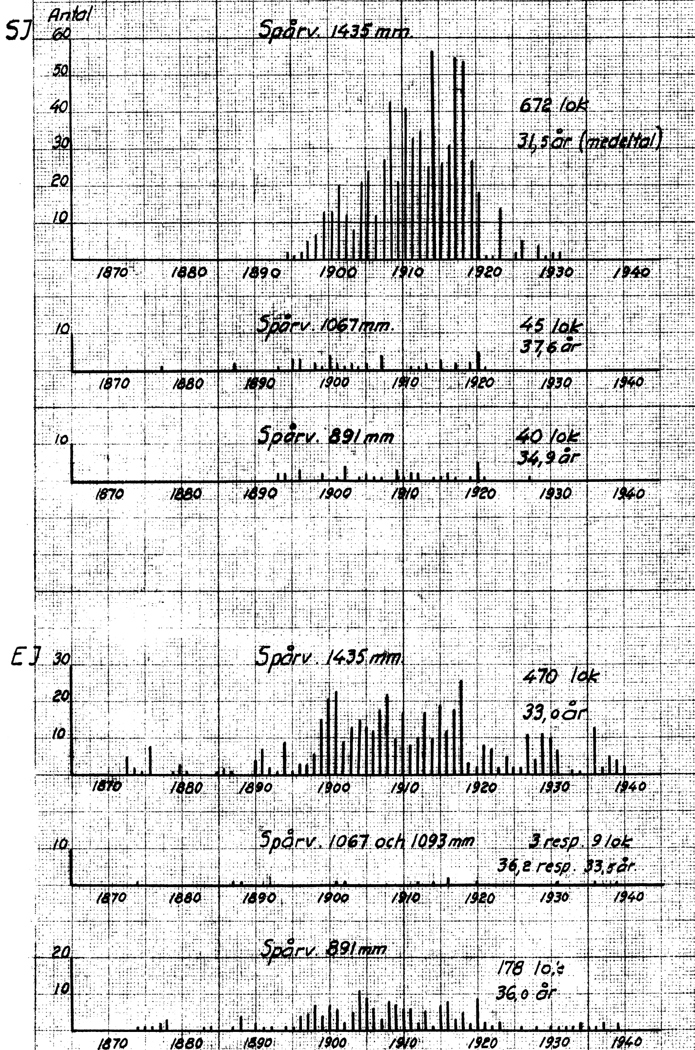
Plansch II. Fördelning av SJ och EJ ånglok efter tillverkningsår
