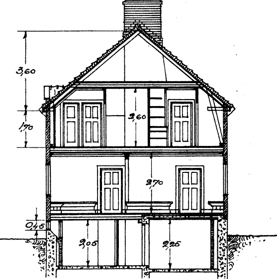
Sektion i A-B
