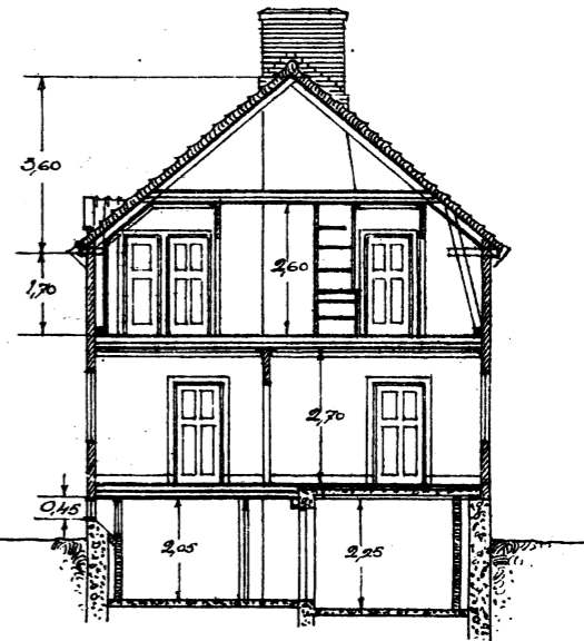
Sektion i A-B.
